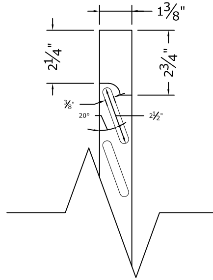
3 Louver Section
