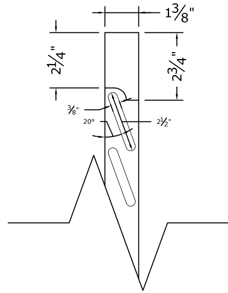
3 Louver Section
