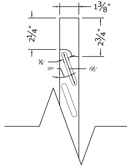
3 Louver Section
