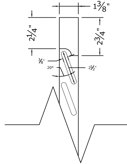
3 Louver Section
